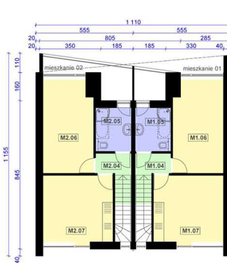
PIĘTRO
